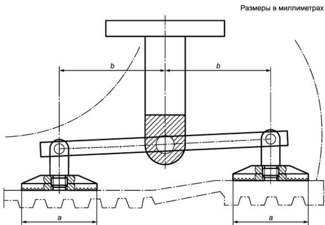
Рисунок А.1 - Пример подходящей механической стопы
